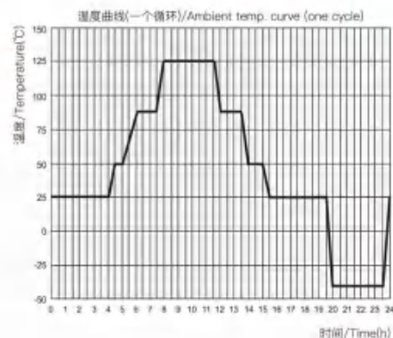
电耐久性试验环境温度曲线
