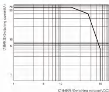
允许最大负载范围(23℃)
