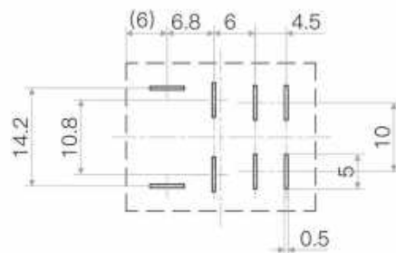
底视图 Bottom view
